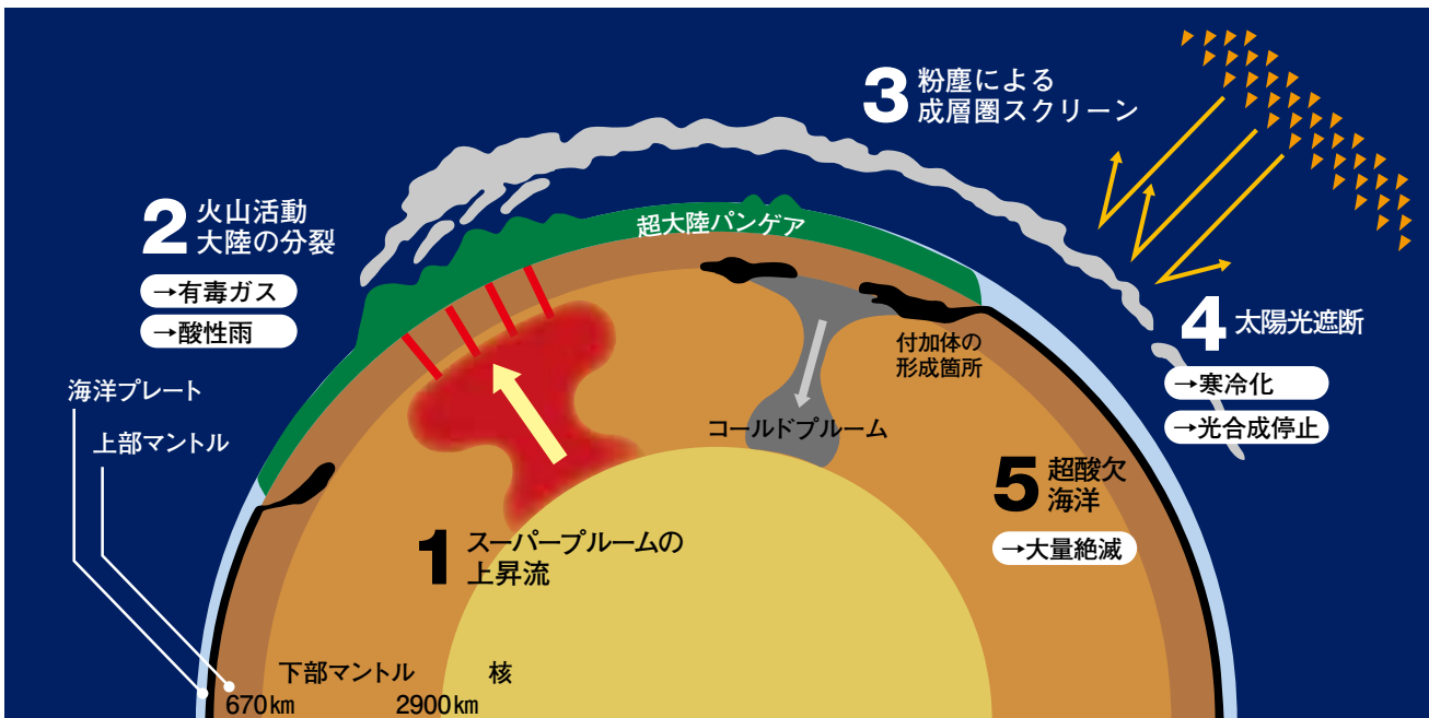
地球内部のマントルにはブルームと呼ぶ大循環があり、その対流変化が結果的に太陽光を遮断し、地表環境の寒冷化によって大量絶滅を起こす。
